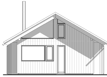
FASADE - ØST
