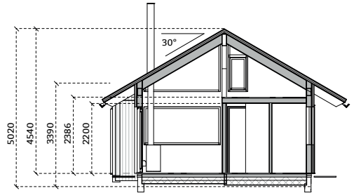
SNITT
