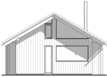
FASADE - VEST
